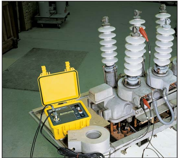
Medición de Razón CT
