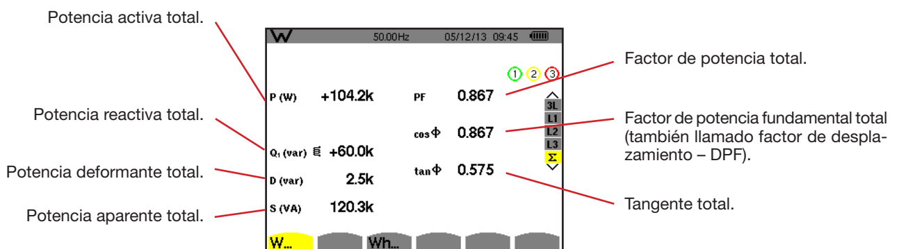
Figura 103: Figura 115: la pantalla de visualización de las potencias y magnitudes totales asociadas en \Sigma
