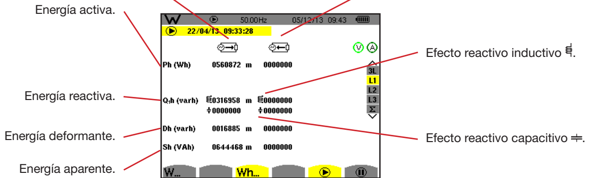
Figura 102: Figura 114: la pantalla de visualización de las energías consumidas y aportadas en L1
