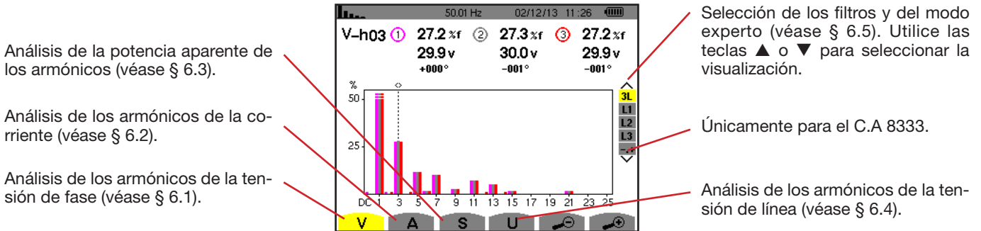
Figura 41: La pantalla del modo armónico
