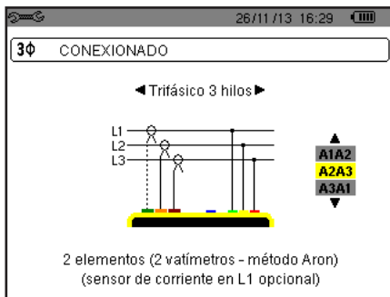
Figura 14: Figura 14: conexión trifásica de 3 hilos
