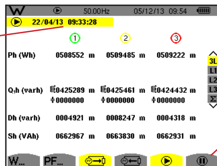
Figura 105: La pantalla de inicio de la medición de energía en Wh
