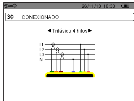
Figura 15: Figura 15: conexión trifásica de 4 hilos
