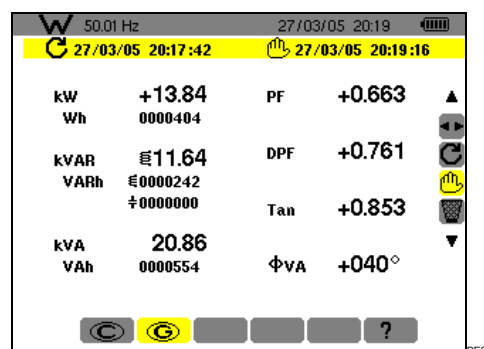
Figura 33: ejemplo de visualización de medidas de potencias y de energías después de un recuento.
