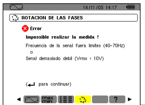
Figura 29: frecuencia fuera de límite o señal demasiado débil.
