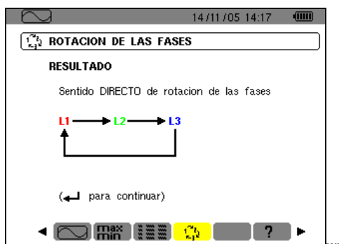
Figura 27: ejemplo del resultado de una medida de un sentido de fases directo.
